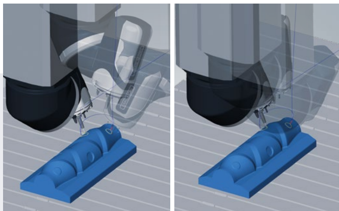
La imagen de la izquierda muestra un gran movimiento del cabezal de la máquina, y la de la derecha muestra el movimiento optimizado
